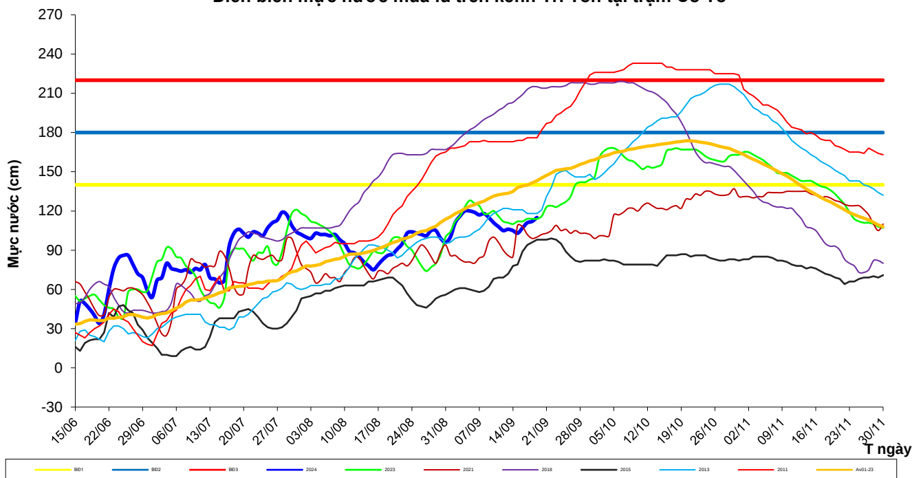
Diễn biến mực nước mùa lũ trên kênh Tri Tôn tại trạm Cỏ Tô
