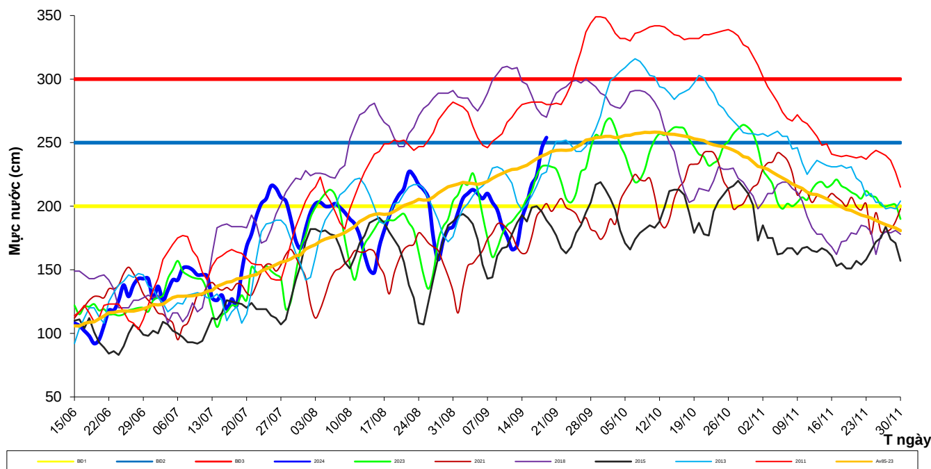
Diễn biến mực nước mùa lũ trên rạch Ông Chường tại trạm Chợ Mới
