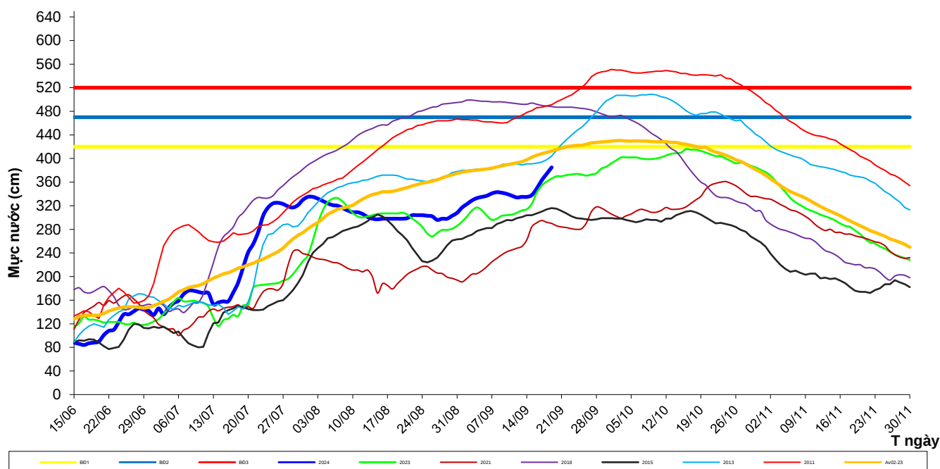
Diễn biến mực nước mùa lũ trên sông Hậu tại trạm Khánh An
