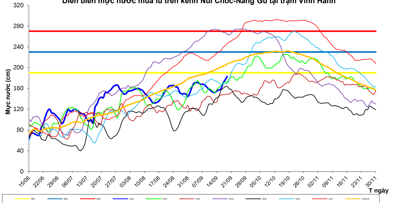
Diễn biến mực nước mùa lũ trên kênh Núi Chóc-Năng Gù tại trạm Vĩnh Hanh
