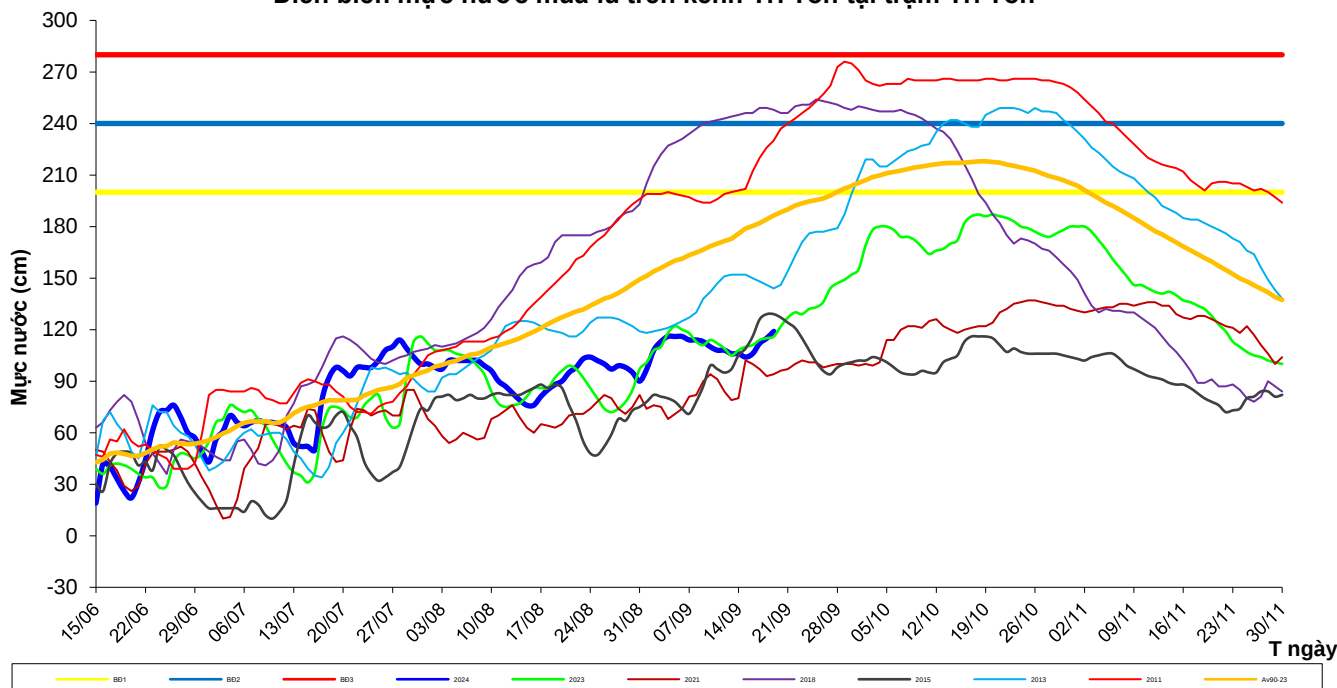
Diễn biến mực nước mùa lũ trên kênh Tri Tôn tại trạm Tri Tôn
