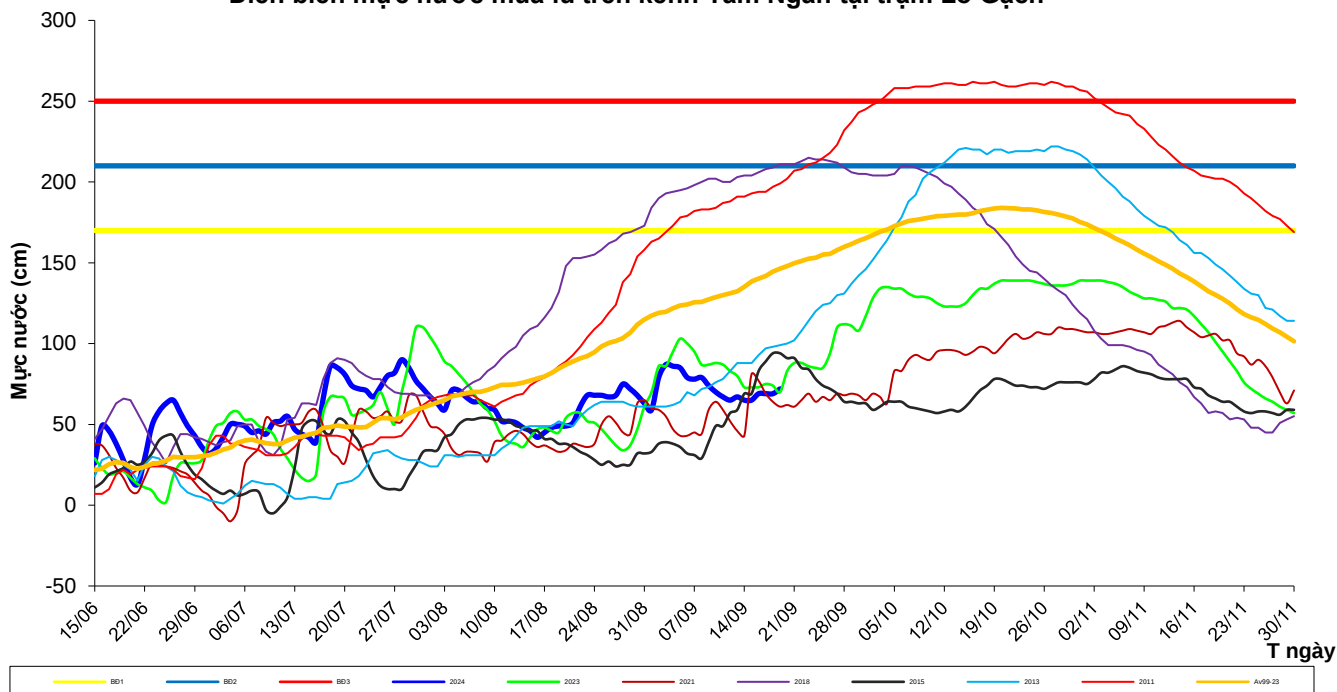
Diễn biến mực nước mùa lũ trên kênh Tám Ngàn tại trạm Lò Gạch
