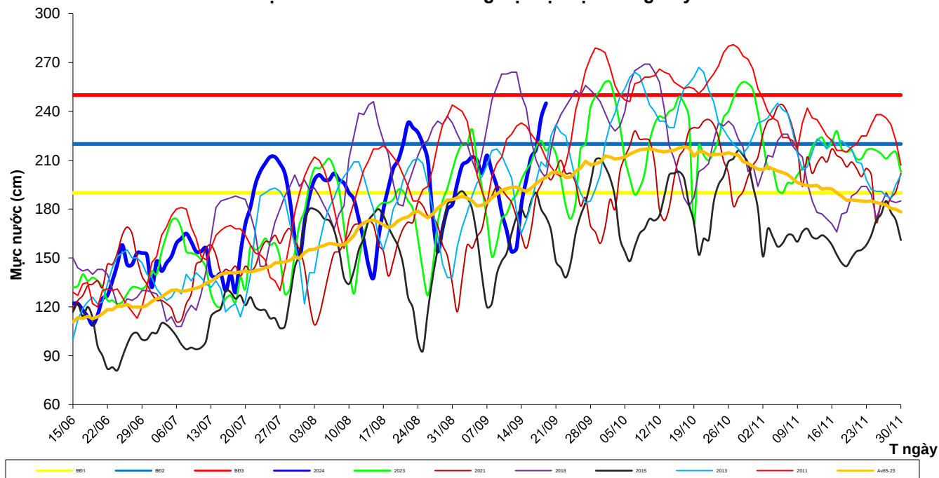
Diễn biến mực nước mùa lũ trên sông Hậu tại trạm Long Xuyên
