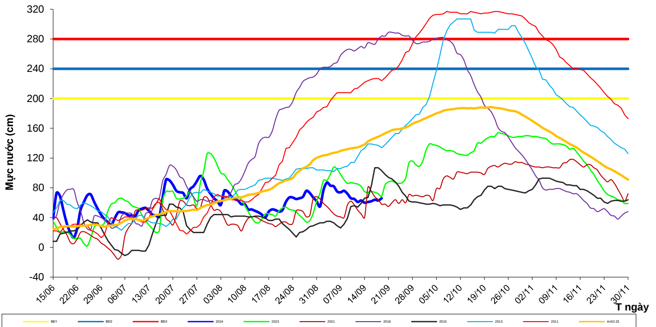
Diễn biến mực nước mùa lũ trên kênh Vĩnh Tế tại trạm Vĩnh Gia
