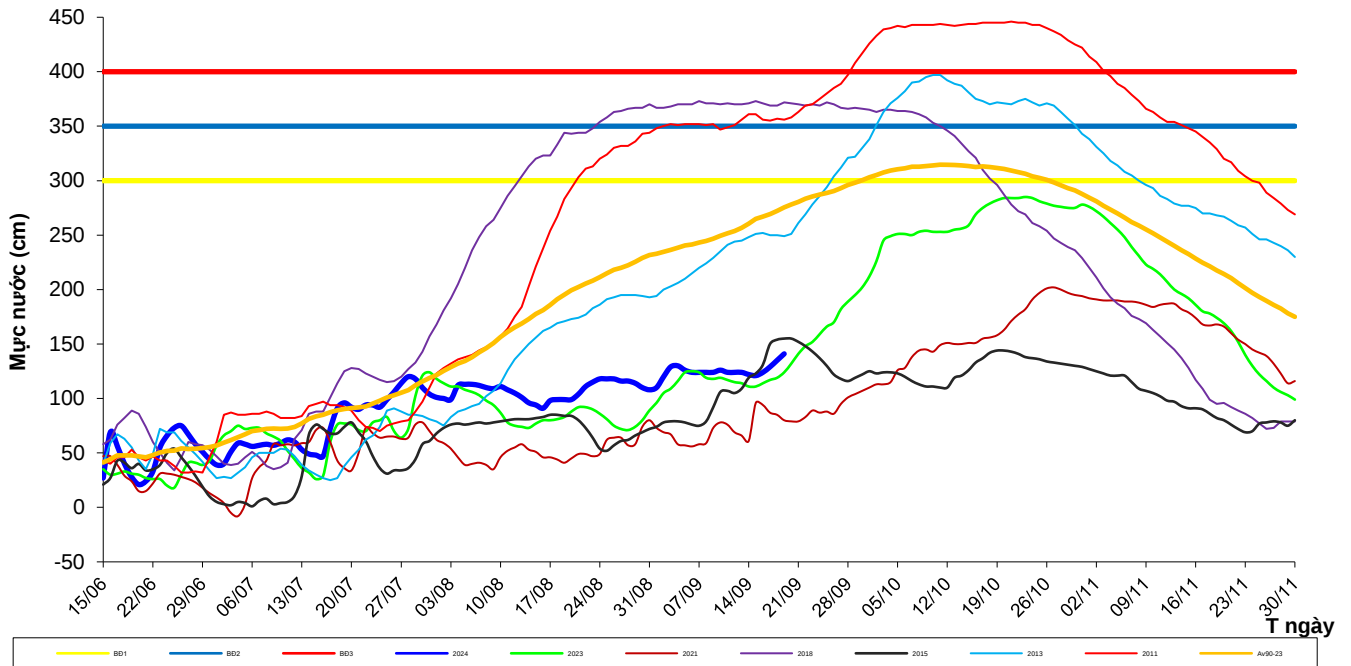
Diễn biến mực nước mùa lũ trên kênh Vĩnh Tế tại trạm Xuân Tô
