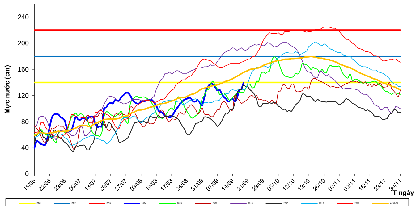
Diễn biến mực nước mùa lũ trên kênh Rạch Giá-Long Xuyên tại trạm Núi Sập
