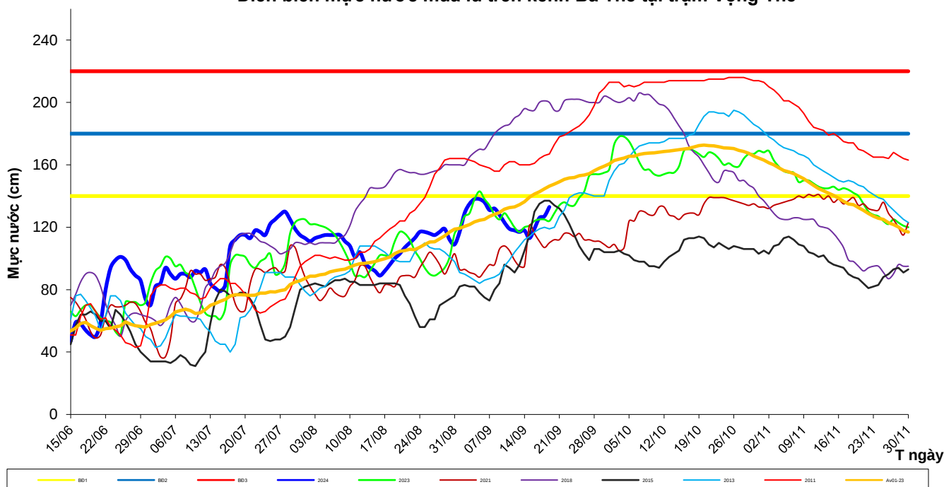
Diễn biến mực nước mùa lũ trên kênh Ba Thê tại trạm Vọng Thê
