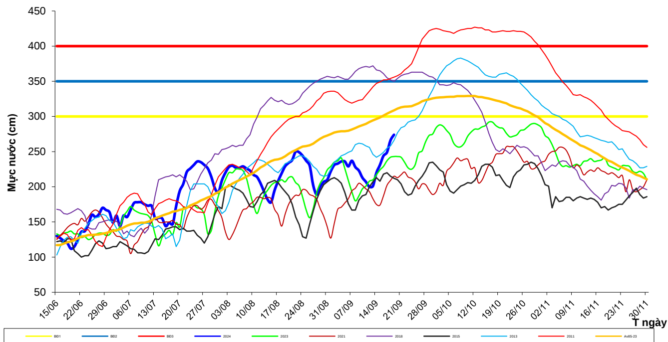
Diễn biến mực nước mùa lũ trên sông Hậu tại trạm Châu Đốc
