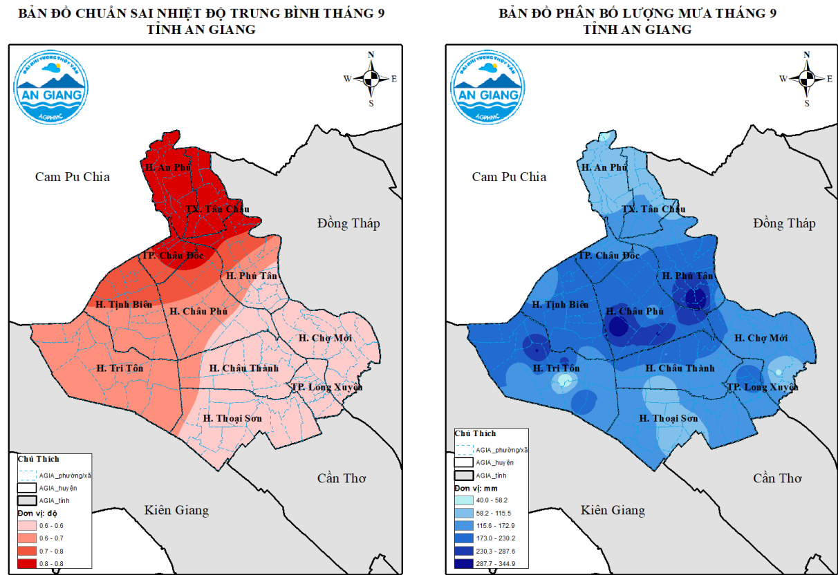
Bản đồ chuẩn sai nhiệt độ trung bình tháng 9/2024 tỉnh An Giang
