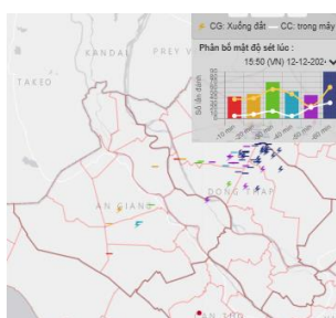
Ảnh định vị sét
