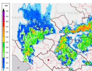
Ảnh Radar thời tiết
