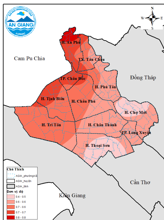
BẢN ĐỒ DỰ BÁO CHUẨN SAI NHIỆT ĐỘ TRUNG BÌNH THÁNG 02 TỈNH AN GIANG
