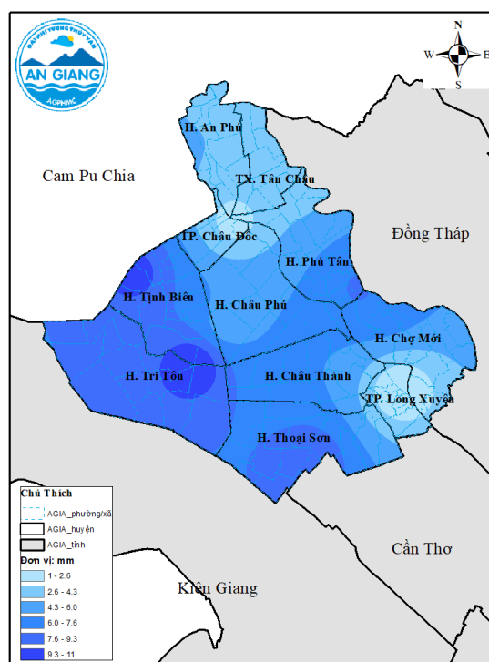
BẢN ĐỒ DỰ BÁO CHUẨN SAI LƯỢNG MƯA THÁNG 02 TỈNH AN GIANG
