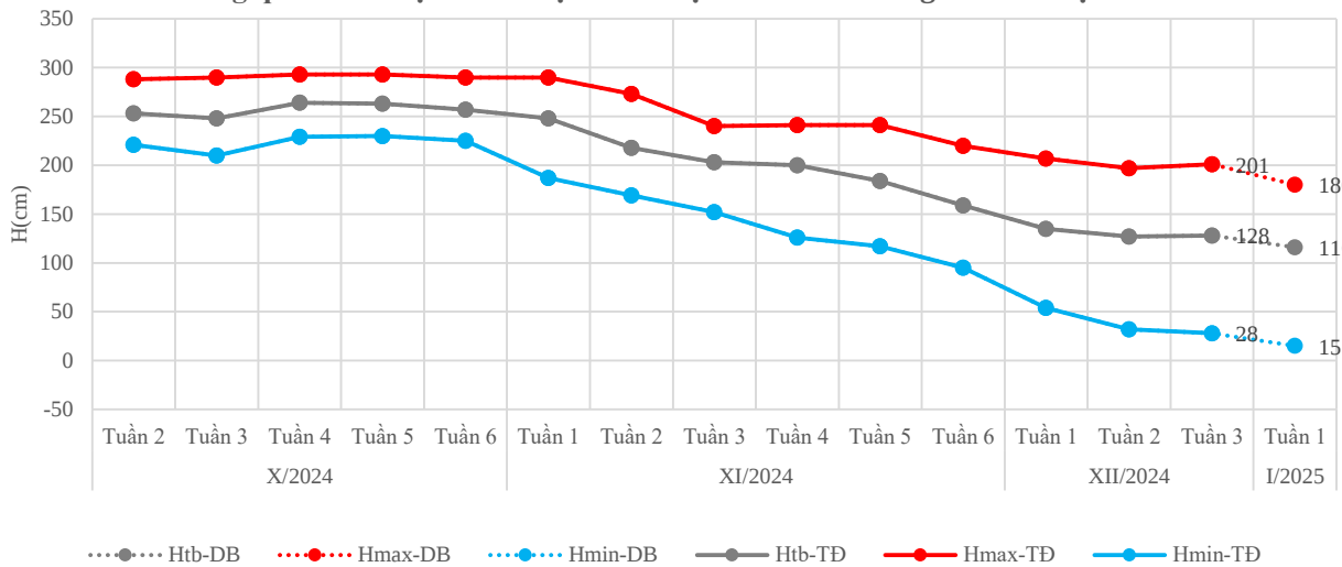
Đường quá trình mực nước thực đo và dự báo tuần 1 tháng 01/2025 trạm Châu Đốc
