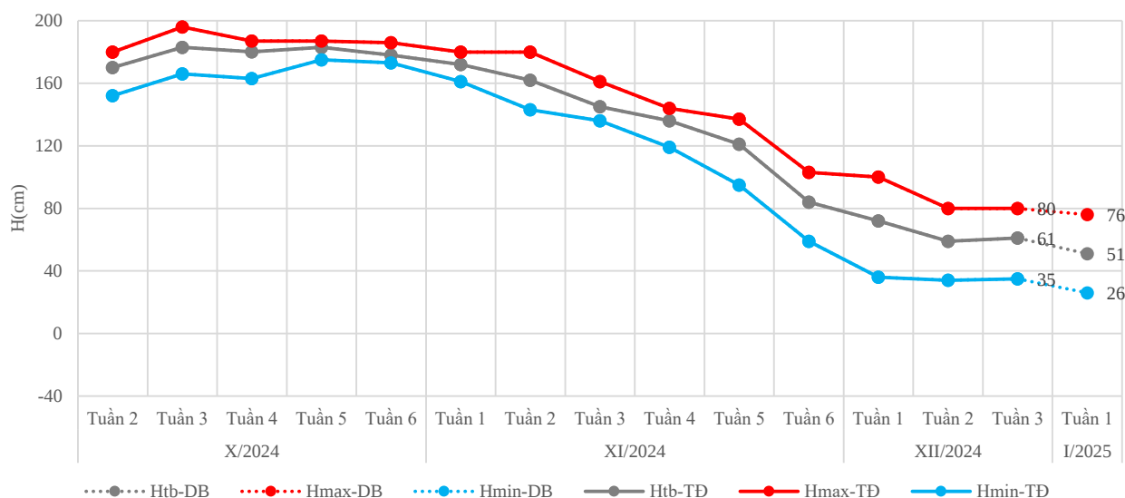
Đường quá trình mực nước thực đo và dự báo tuần 1 tháng 01/2025 trạm Tri Tôn
