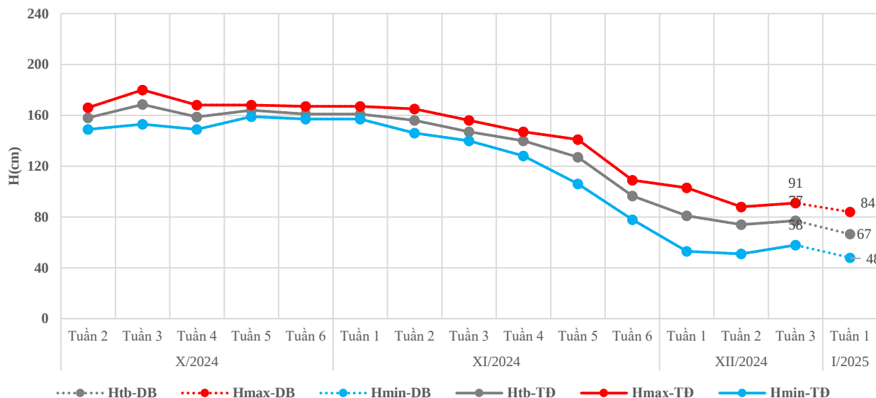
Đường quá trình mực nước thực đo và dự báo tuần 1 tháng 1/2025 trạm Cồ Tô
