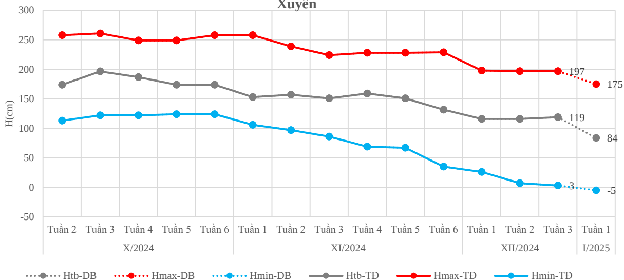
Đường quá trình mực nước thực đo và dự báo tuần 1 tháng 01/2025 trạm Long Xuyên
