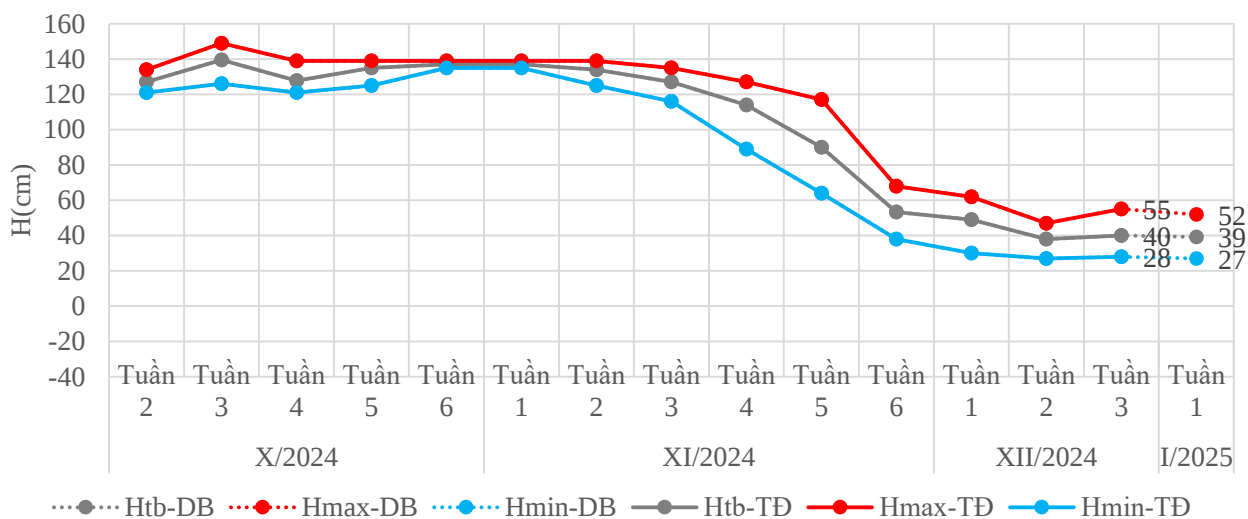
Đường quá trình mực nước thực đo và dự báo tuần 1 tháng 01/2025 trạm Lò Gạch
