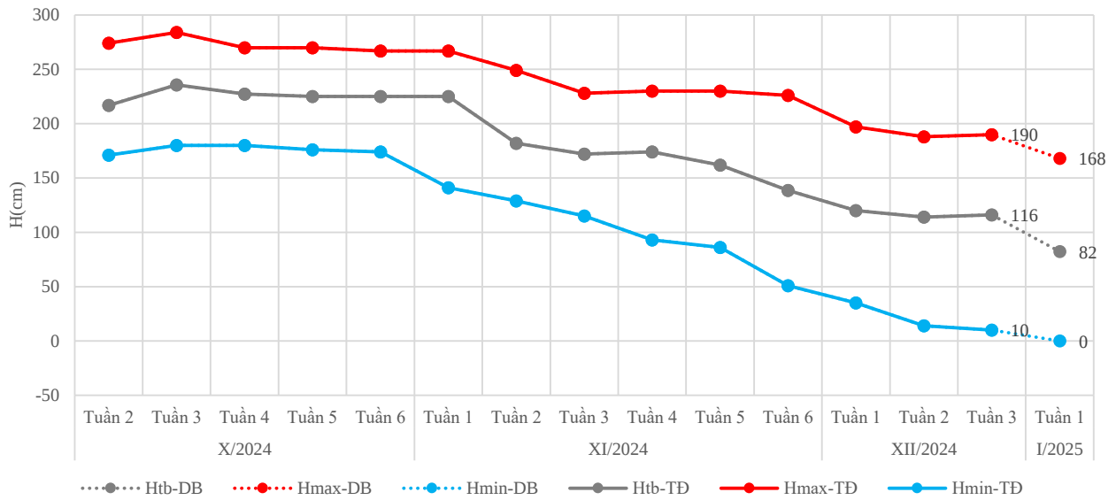
Đường quá trình mực nước thực đo và dự báo tuần 1 tháng 01/2025 trạm Vàm Nao
