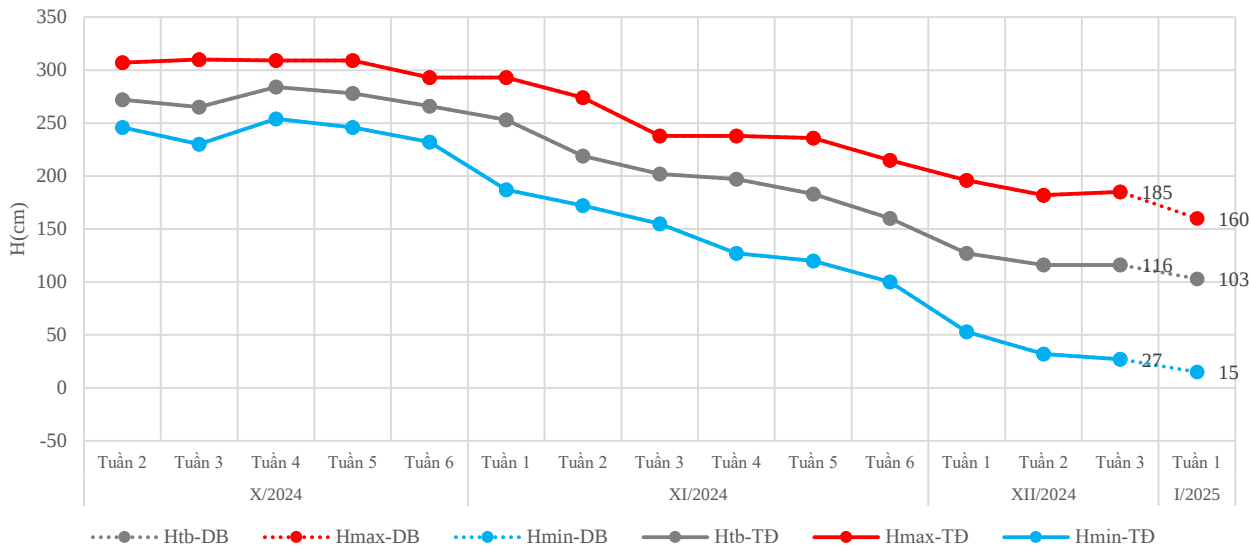
Đường quá trình mực nước thực đo và dự báo tuần 1 tháng 01/2025 trạm Tân Châu
