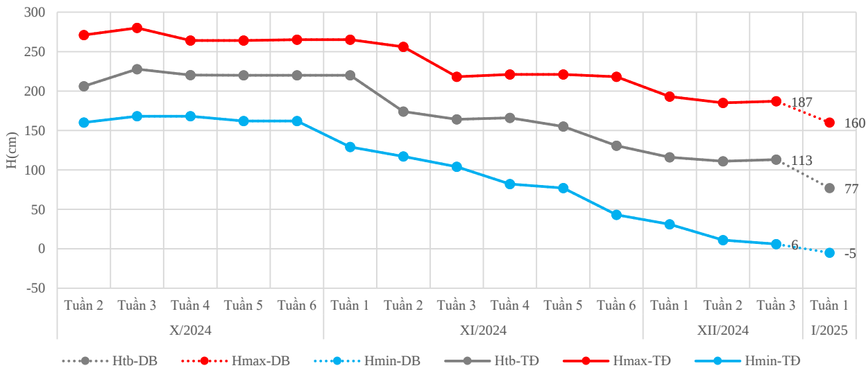
Đường quá trình mực nước thực đo và dự báo tuần 1 tháng 01/2025 trạm Chợ Mới
