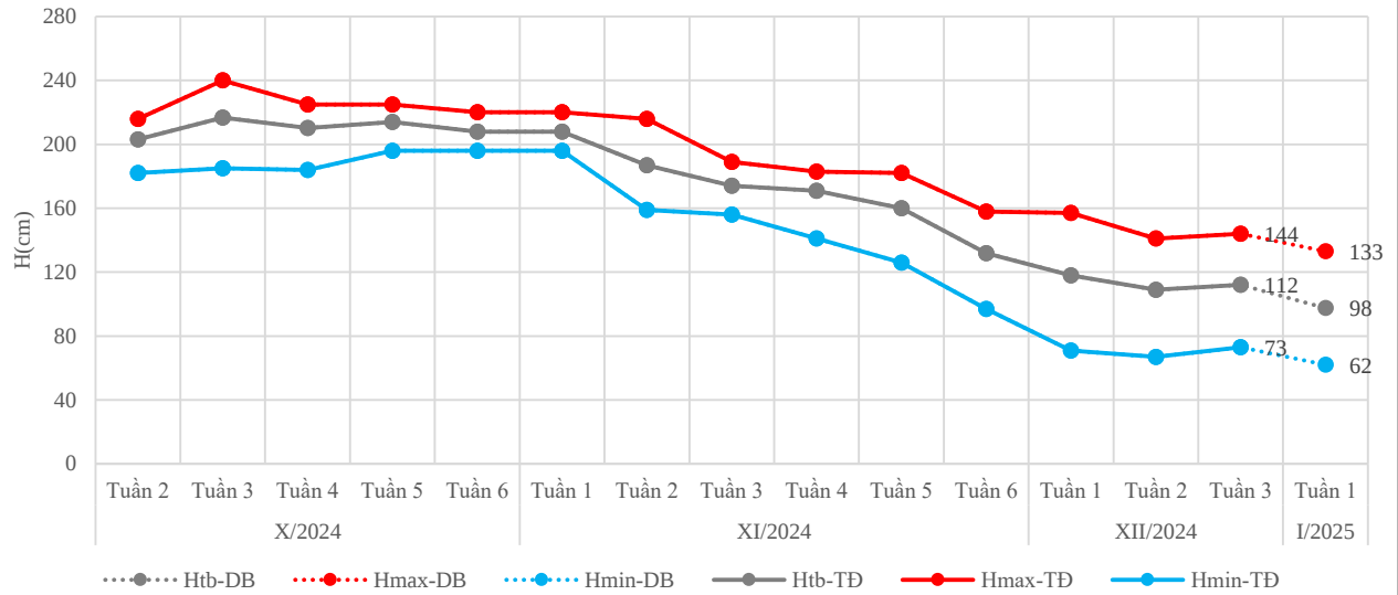
Đường quá trình mực nước thực đo và dự báo tuần 1 tháng 01/2025 trạm Vĩnh Hạnh
