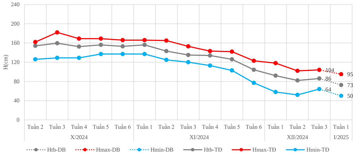
Đường quá trình mực nước thực đo và dự báo tuần 1 tháng 01/2025 trạm Núi Sập
