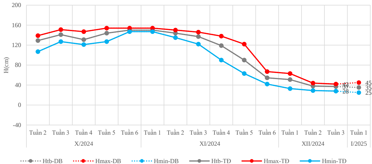
Đường quá trình mực nước thực đo và dự báo tuần 1 tháng 01/2025 trạm Vĩnh Gia
