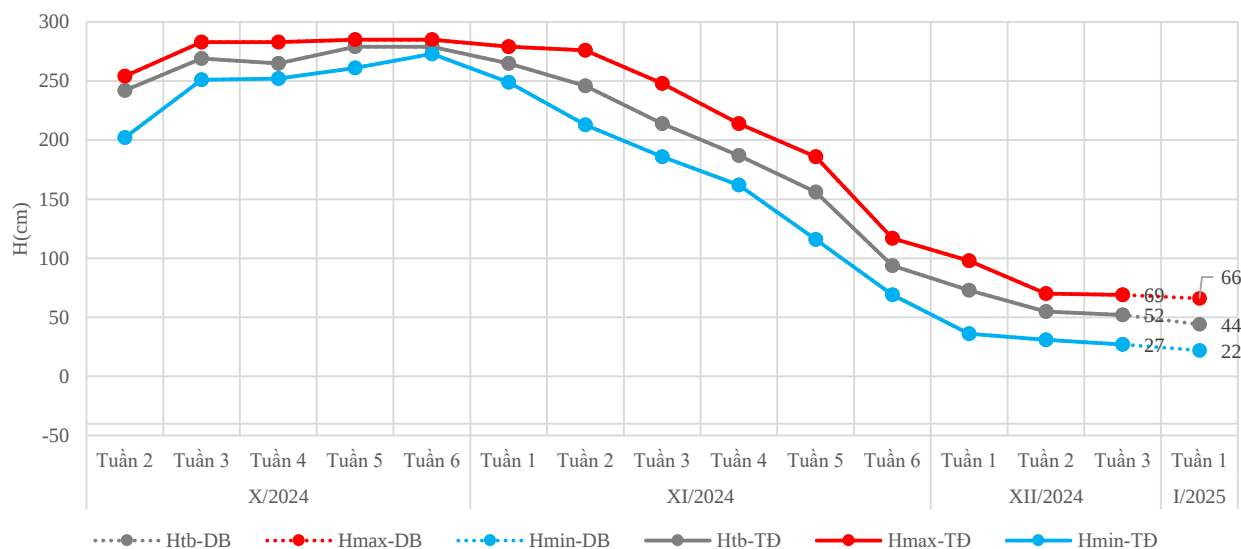
Đường quá trình mực nước thực đo và dự báo tuần 1 tháng 01/2025 trạm Xuân Tô
