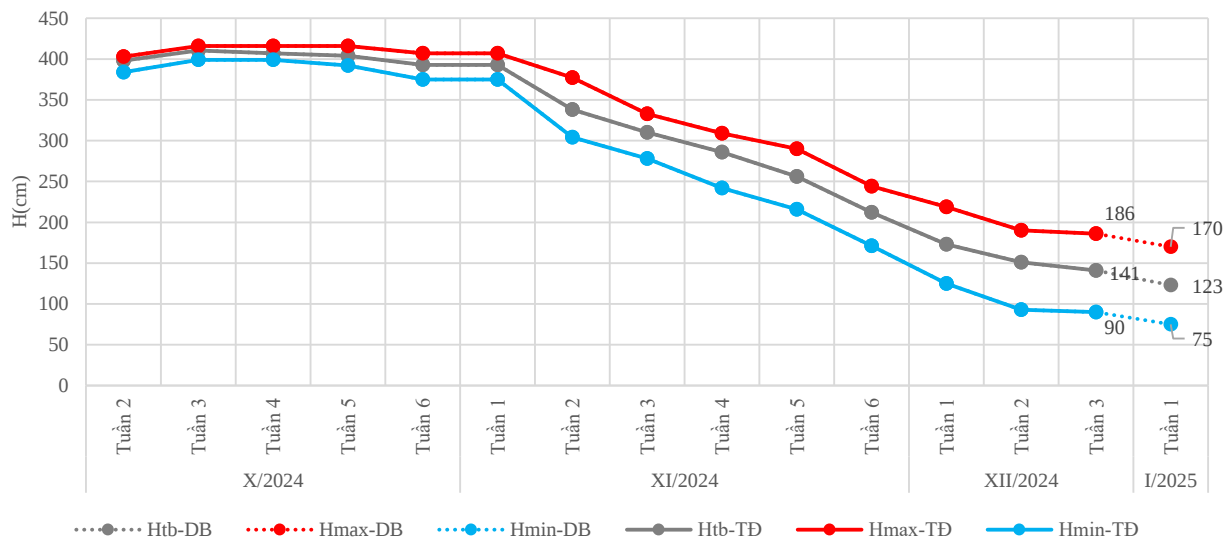
Đường quá trình mực nước thực đo và dự báo tuần 1 tháng 01/2025 trạm Khánh An
