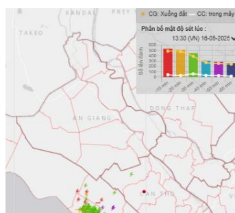
Ảnh định vị sét
