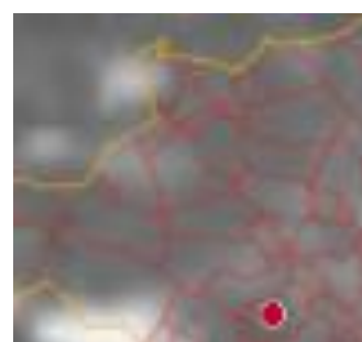
Ảnh mây vệ tinh
