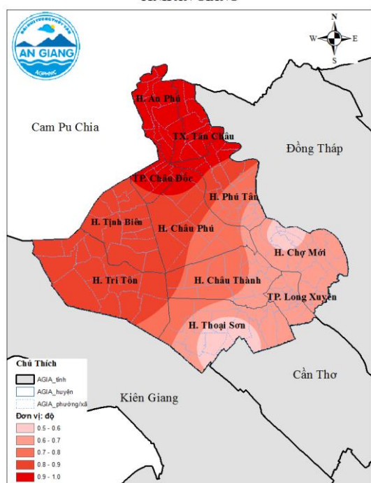
BẢN ĐỒ DỰ BÁO CHUẨN NHIỆT ĐỘ TRUNG BÌNH THÁNG 6 TỈNH AN GIANG
