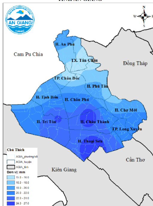
BẢN ĐỒ CHUẨN SAI LƯỢNG MƯA THÁNG 6 TỈNH AN GIANG
