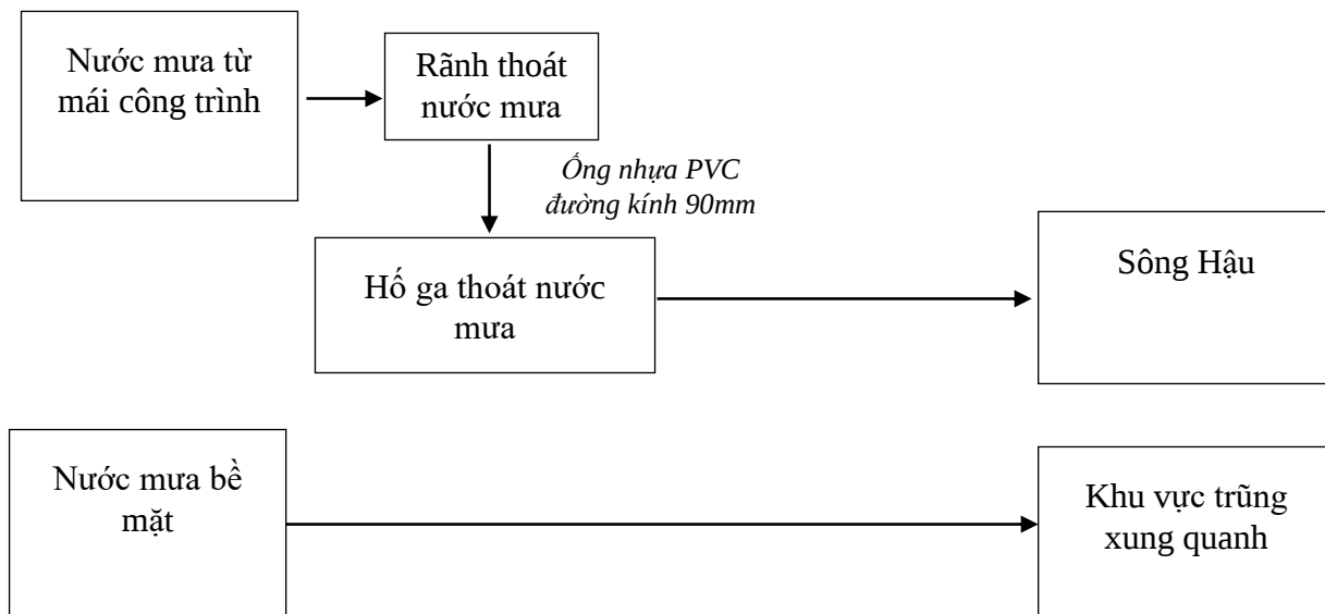
Hình 4. Sơ đồ thu gom, thoát nước mưa
