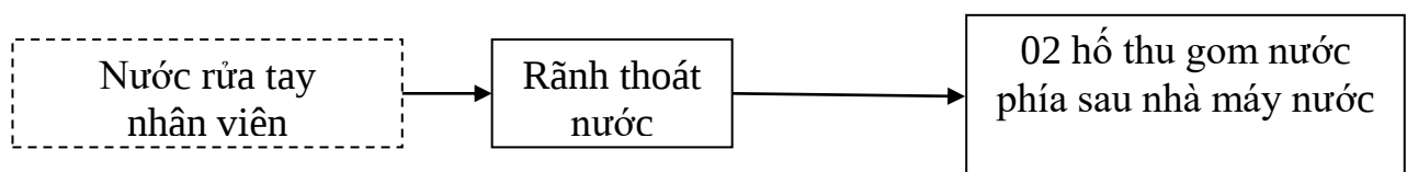
Hình 6. Sơ đồ thu gom và thoát nước rửa tay nhân viên
